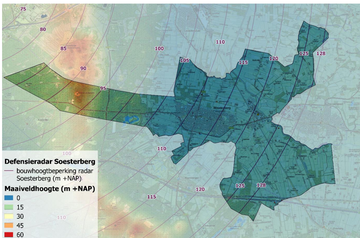
Figuur 7: Defensieradar Soesterberg - bouwhoogtebeperking
