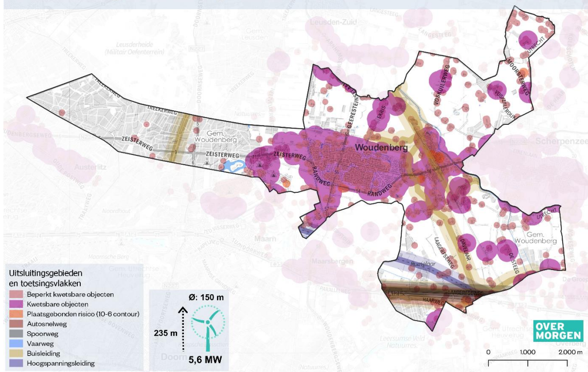
Figuur 6: Belemmeringen windenergie 5,6 MW
